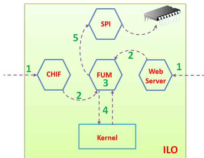
شکل ۵- فرآیند به‌روزرسانی سفت‌افزار iLO توسط ماژول FUM
