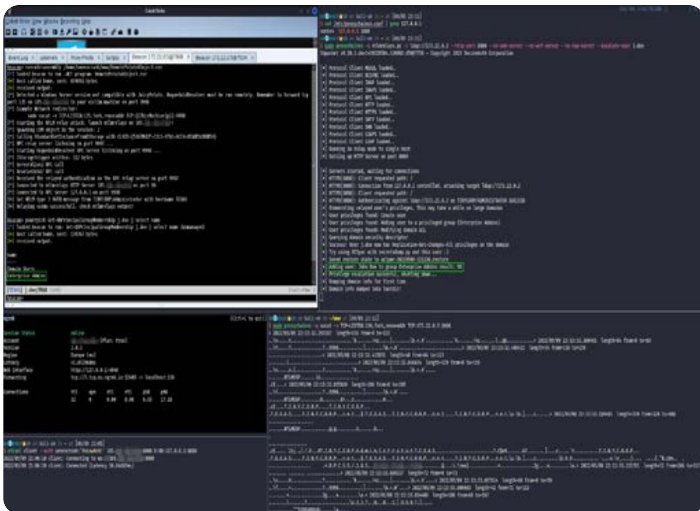
Рис. 19. Релеим НТТР через chisel
