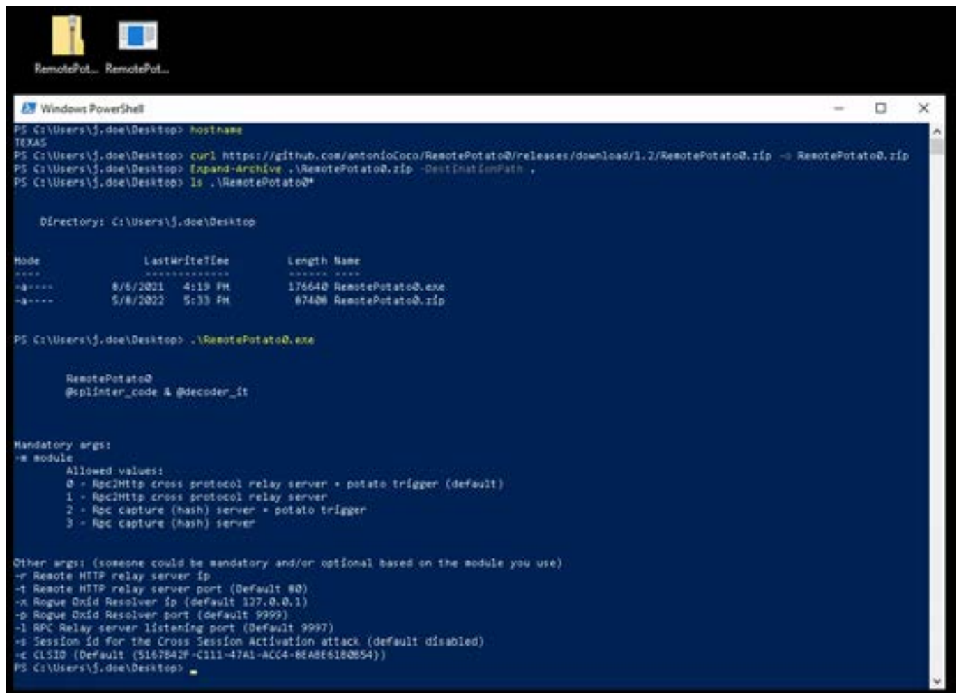
Рис. 8. Загрузка и распаковка RemotePotato0
